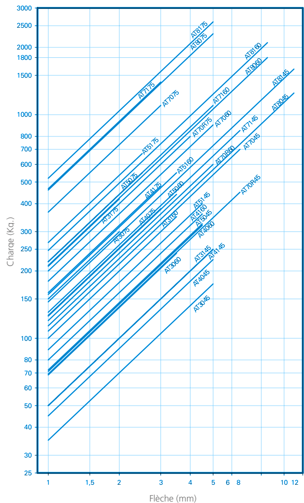
COURBE DE CHARGE-FLÈCHE AMC MECANOCAUCHO® TYPE AT 30-81
