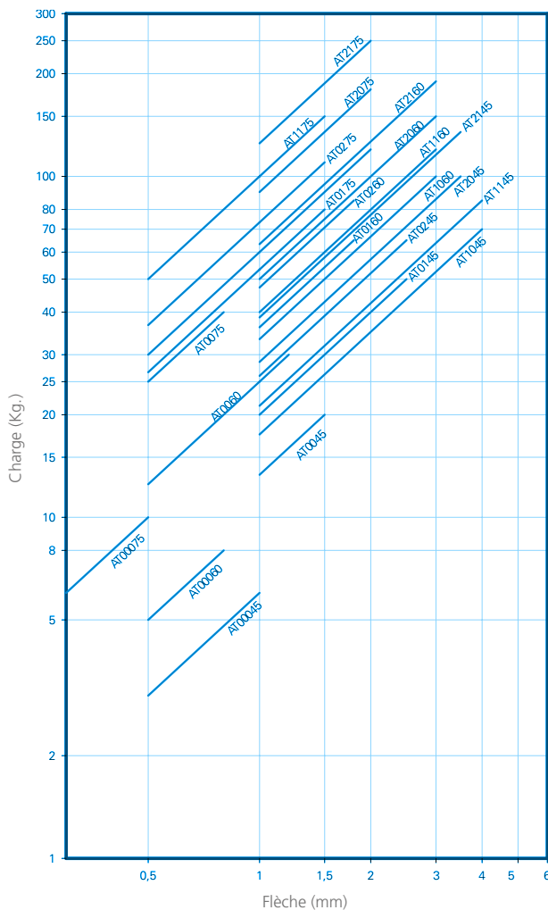
COURBE DE CHARGE-FLÈCHE AMC MECANOCAUCHO® TYPE AT 000-21
