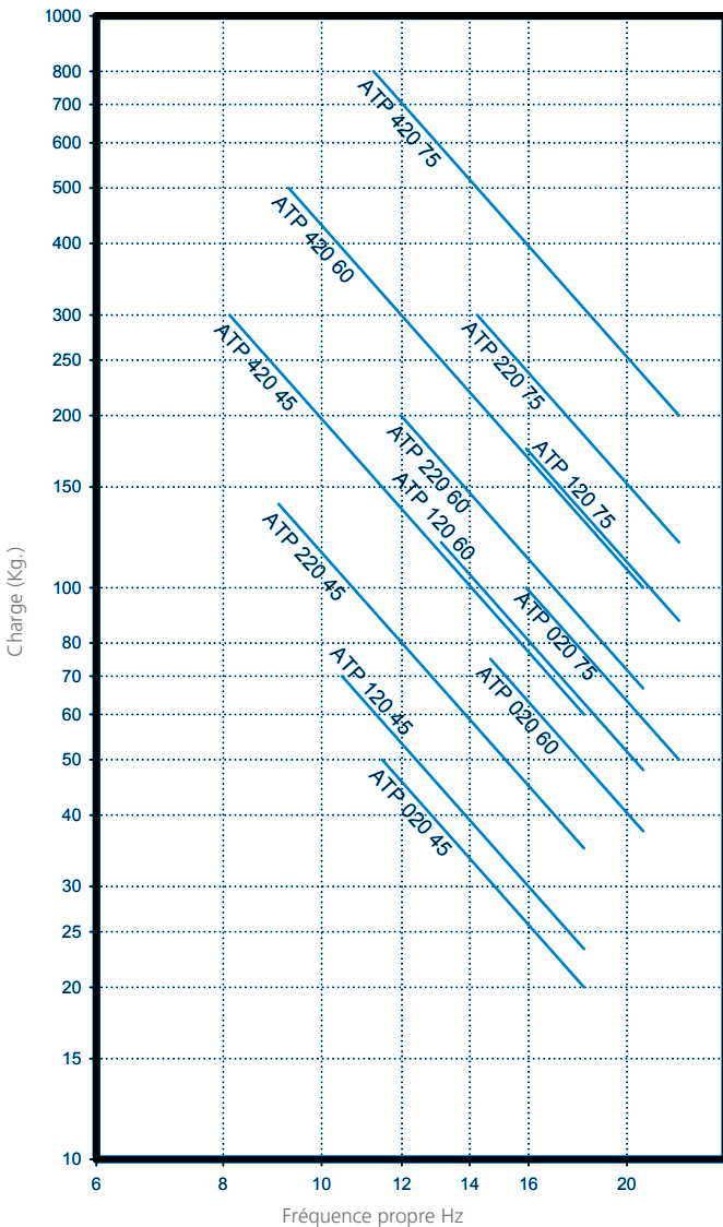
FRÉQUENCE PROPRE AMC MECANOCAUCHO® TYPE ATP
