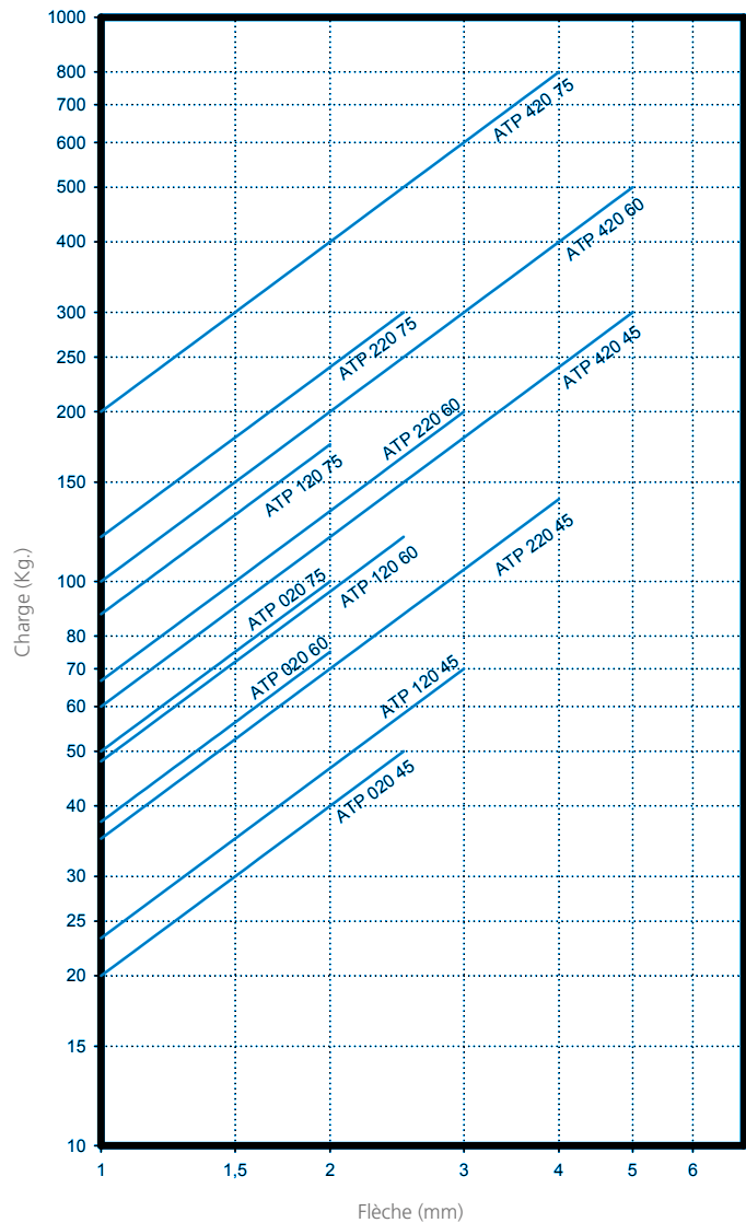
COURBE DE CHARGE-FLÈCHE AMC MECANOCAUCHO® TYPE ATP
