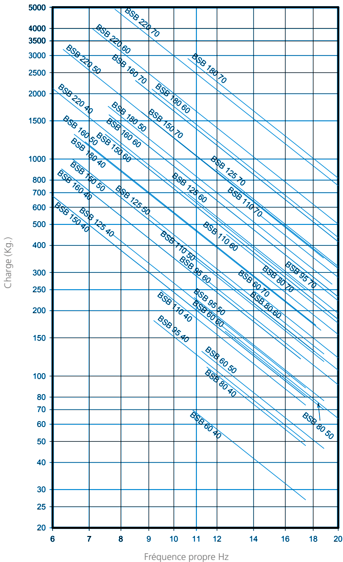
FRÉQUENCE PROPRE AMC MECANOCAUCHO® TYPE BSB
