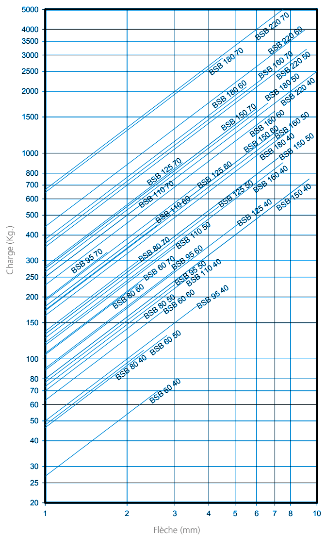
COURBE DE CHARGE-FLÈCHE AMC MECANOCAUCHO® TYPE BSB
